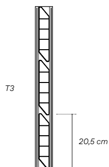
VISTA INTERIOR Poste Vall Vent Plus
