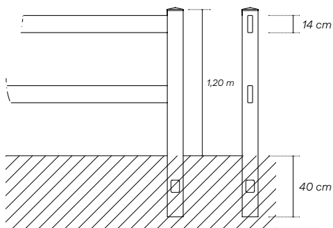
VISTA FRONTAL Cercado Post-Rail de 1,2 m.
