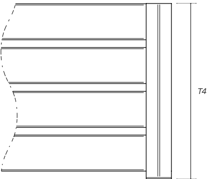
VISTA FRONTAL Vall Palau Ventilado 3 cm
