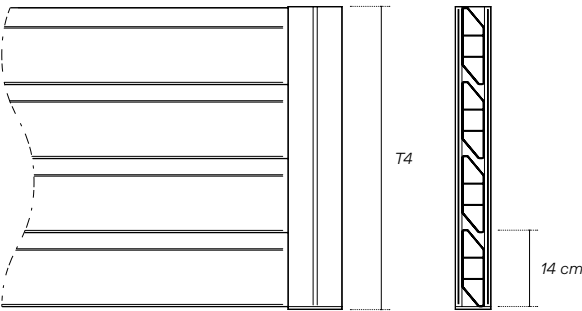
VISTA FRONTAL Vall Vent estándar
