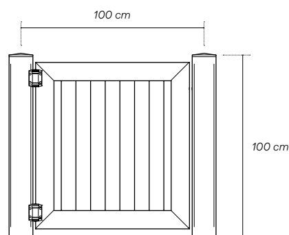
VISTA FRONTAL Puerta Valla de Piscina Ágata
