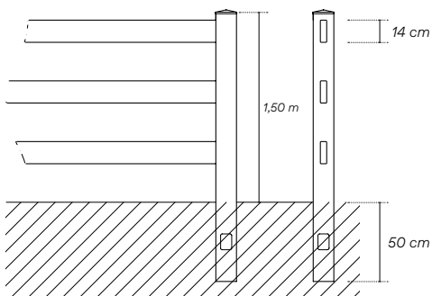
VISTA FRONTAL Cercado Post-Rail de 1,5 m.
