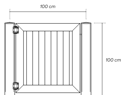
VISTA FRONTAL Puerta Valla de Piscina Rubí
